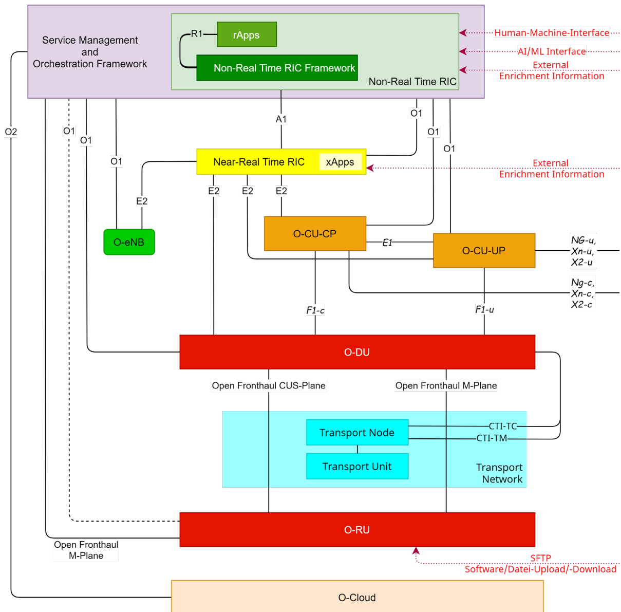
Abbildung 10: O-RAN-Schnittstellen
