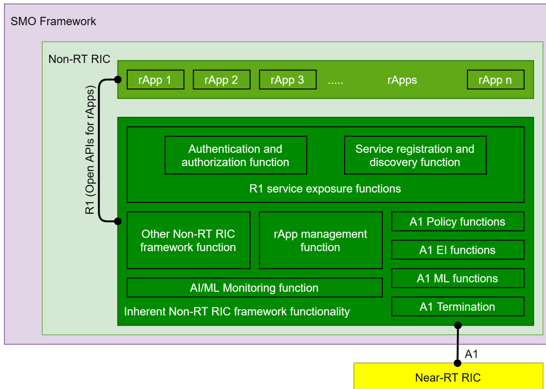
Abbildung 16: Illustration der R1-Schnittstelle über das funktionale Diagramm der Non-RT RIC-Architektur (Ref. [28])
