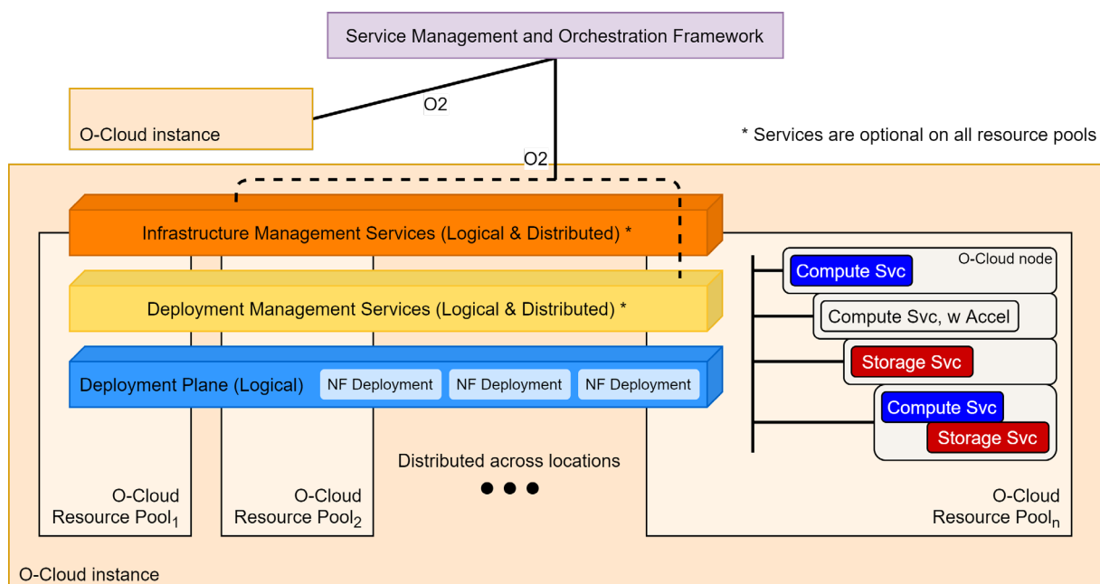
Abbildung 14: Zusammenspiel zwischen SMO-Framework und O-Cloud-Instanzen sowie Übersicht zu den O-Cloud-Kernkomponenten (Ref. [26])
