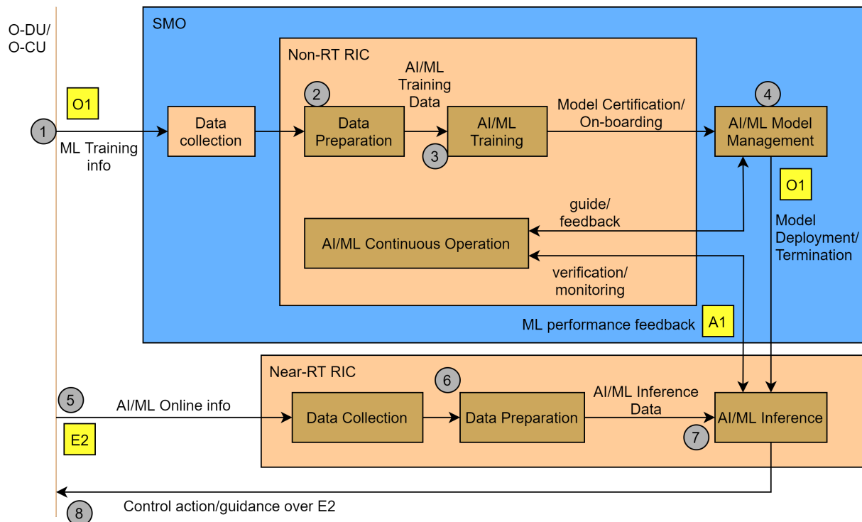
Abbildung 22: Deployment-Szenario für AI/ML [34]
