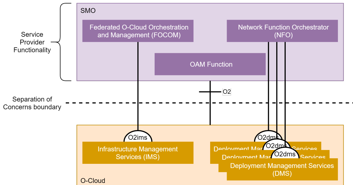
Abbildung 13: Aufteilung der O2-Schnittstelle in Service Based Interfaces (Ref. [25])
