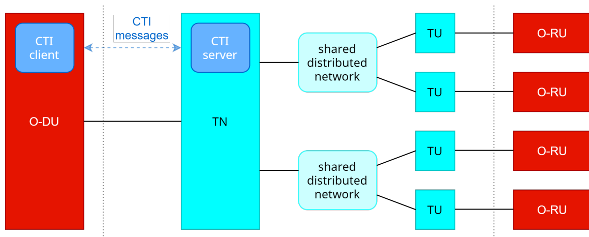
Abbildung 20: Zusammenhang zwischen CTI und dem für das Fronthaul verwendete Transportnetz (Ref. [32])
